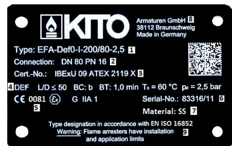
Beispiel Typenschild
