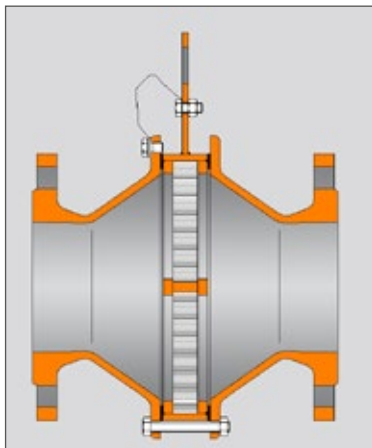
Рис. 13: Противодефлаграционный предохранитель KITO®
