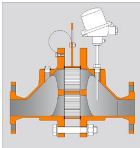
Рис. 14: Противодефлаграционный предохранитель KITO®, эксцентрическая конструкция
