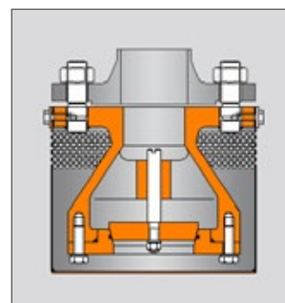
Рис. 9: Обратный клапан KITO®
