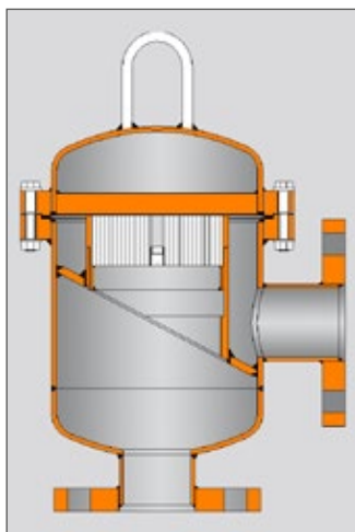
Рис. 10: Противодетонационный преградитель KITO® угловой формы
