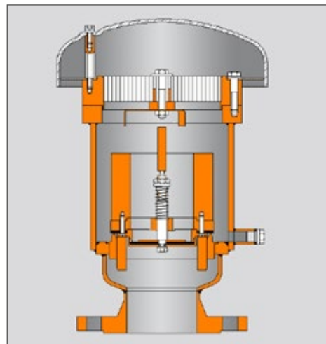
Рис. 5: Комбинированный быстродействующий компенсационный клапан КИТО® для избыточного/пониженного давления
