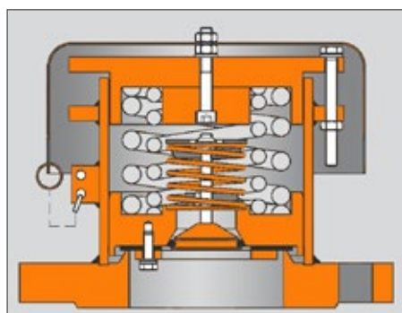
Рис. 17: Клапан KITO® для вагона-цистерны
