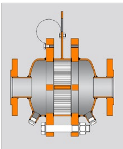
Рис. 6: Противодетонационный преградитель KITO®
