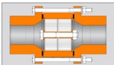
Рис. 16: Противодефлаграционный предохранитель KITO®
