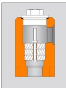
Рис. 7: Противодетонационный преградитель KITO®
