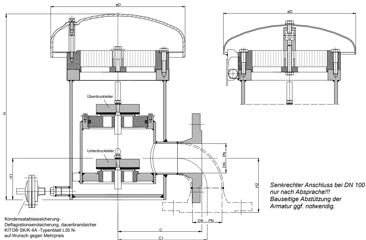
KITO® VD/KL-IIA-...-A
